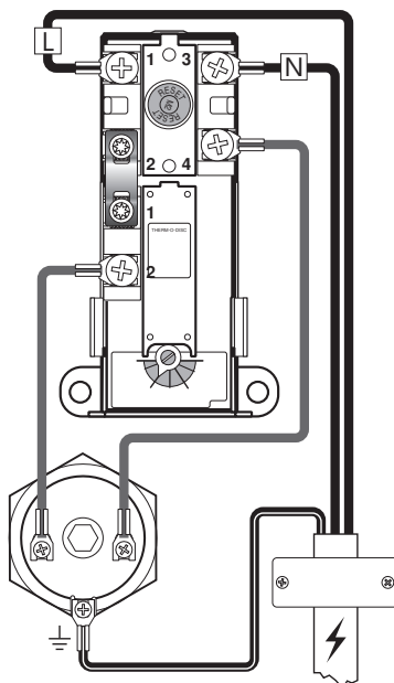
KytKentäkaavio - 3 kW - 1x230V Yläsäiliön normaalikytKentä
