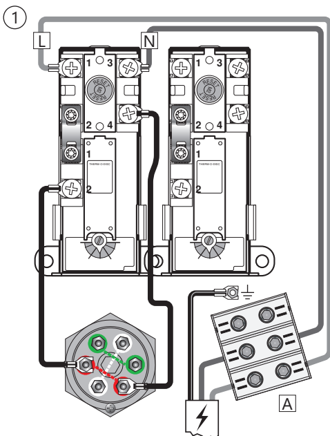
KytKentäkaavio - 3 kW - 2x230V Alasäiliön vaihtoehtoinen kytKentä
