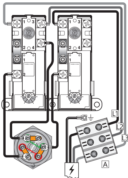
KytKentäkaavio - 9 kW - 3x230V Aläsäiliön normaalikytKentä
