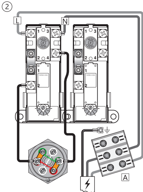
KytKentäkaavio - 6 kW - 2x230V Alasäiliön vaihtoehtoinen kytKentä
