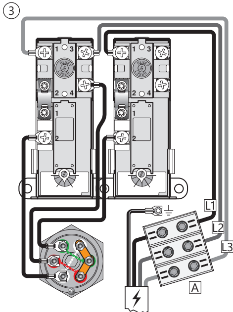
KytKentäkaavio - 9 kW - 3x400V Alasäiliön vaihtoeht. kytKentä - HUOM Nollajohdin EI OLE mahdollinen.
