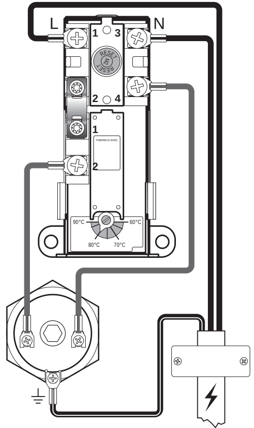
Kytkenäkaavio
